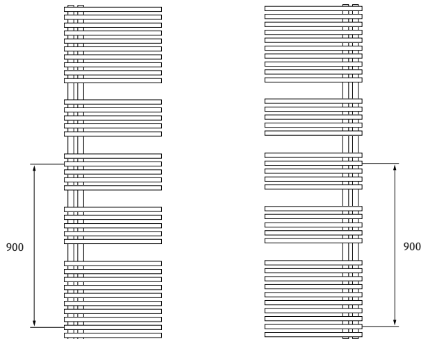
Ausführung links (seitlicher Anschluss links/rechts offen) Ausführung rechts (seitlicher Anschluss rechts/links offen)
