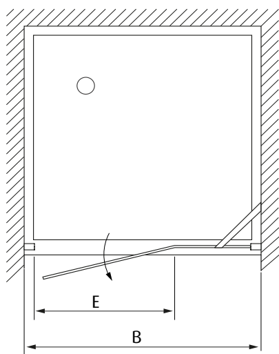
Türelement Anschlag rechts
